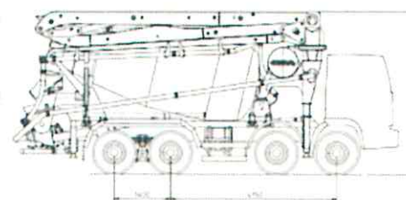
Схема раскладки автобетононасоса
