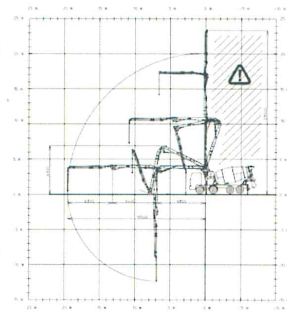
Схема раскладки автобетононасоса
